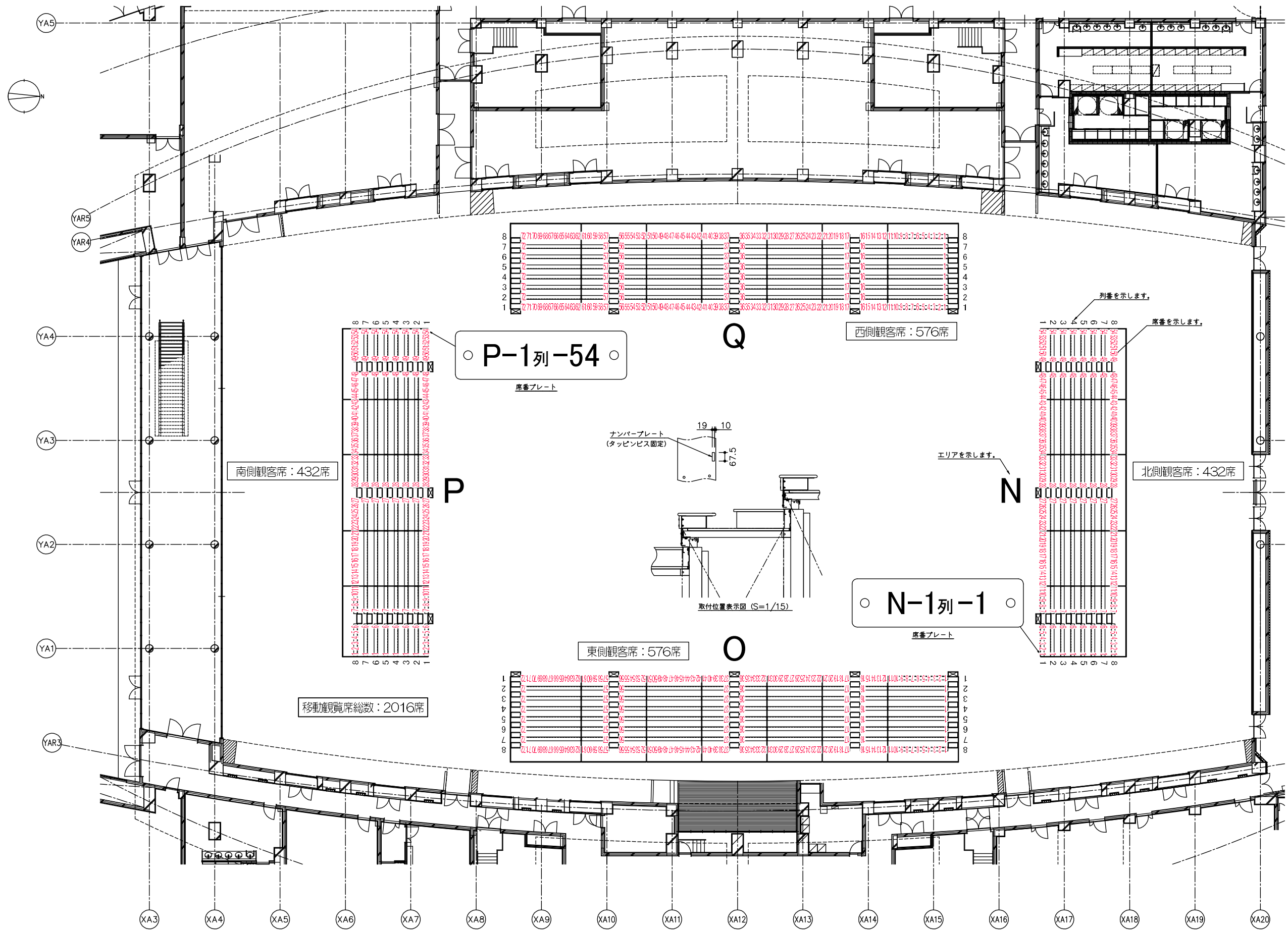
1F 移動観覧席 席番割付図
